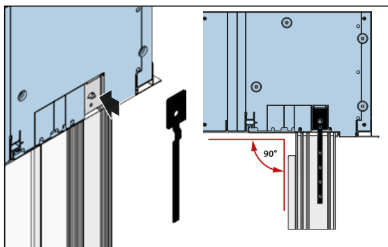
Abbildung 5: verzinkte Rahmenanker
