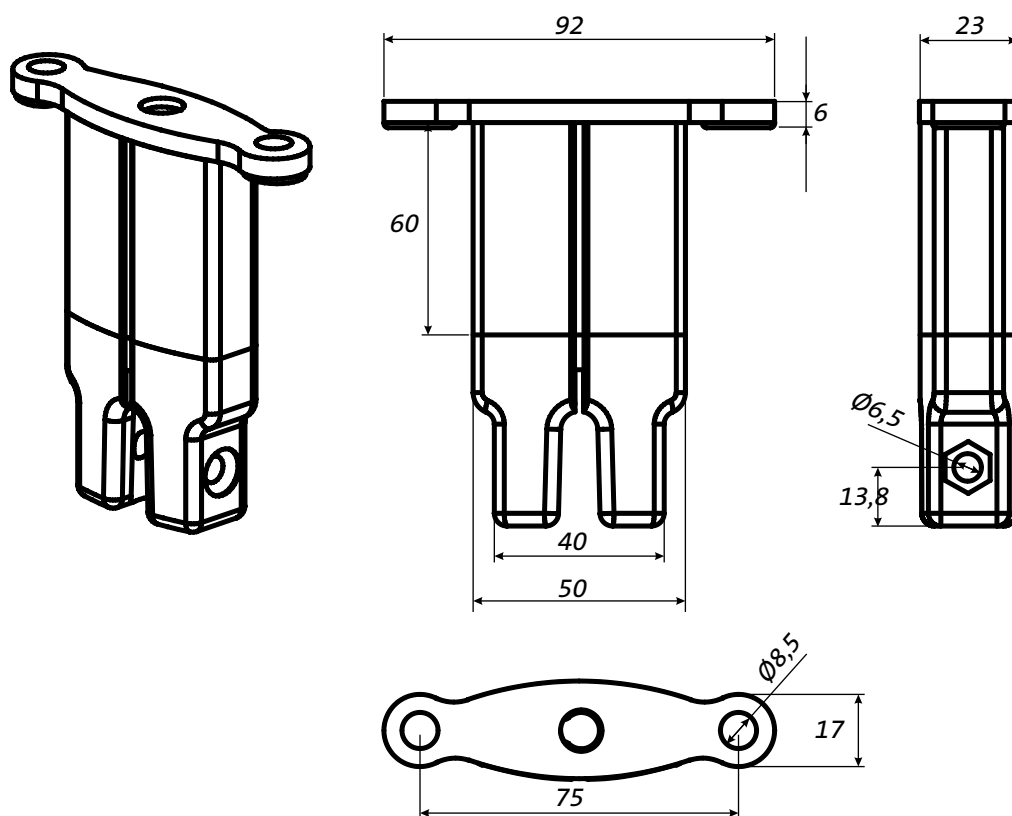
Verhoogde steun Alu. (Standaard)
