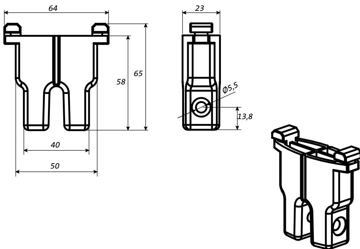
Steun bovendeel (kunststof)
