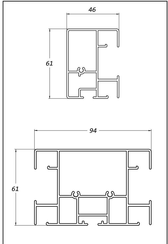
Fig. 1 : Guides
