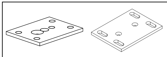
Fig. 11 & 12 : Coupling plates
