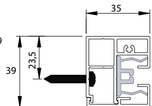
Schiene 803: Standard-Führungsschiene für den Montagetyp 1
