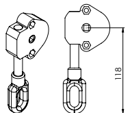
Kegelradgetriebe mit Öse
