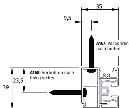
Standard Seitenführungsschiene 801 für Montagetyp 1 (MT1)
