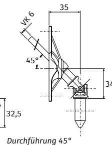
Durchführung 45°
