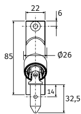
Durchführung 90°
