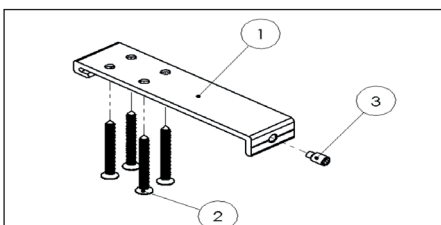
Fig. 30: Montagebeugel
