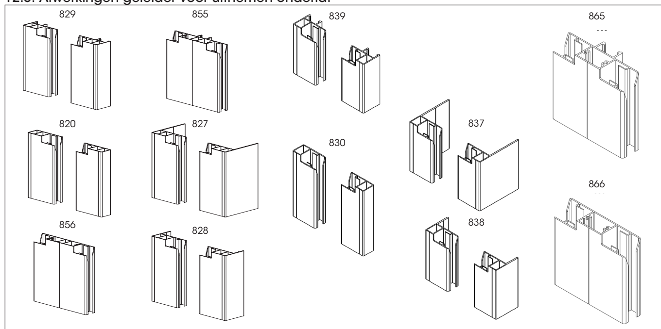
Fig. 23: Standaard afwerking zijgeleiders en middengeleiders
