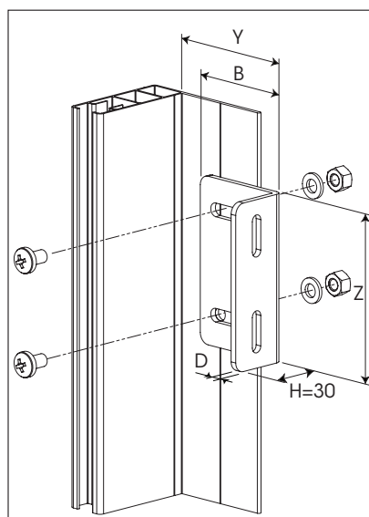
Fig. 22: Afstandsteun
