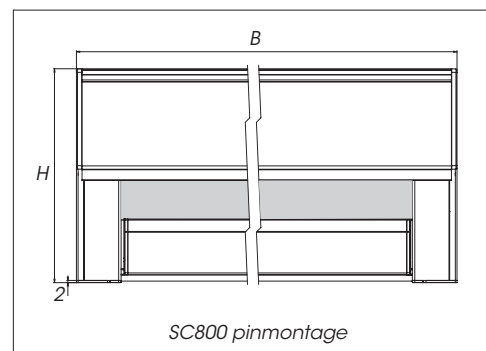
Fig. 3: Afgewerkte maten
