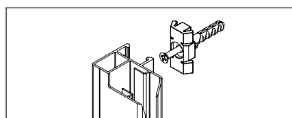
Fig. 20: Clipjes voor geleider 829, 856, 839 en 865
