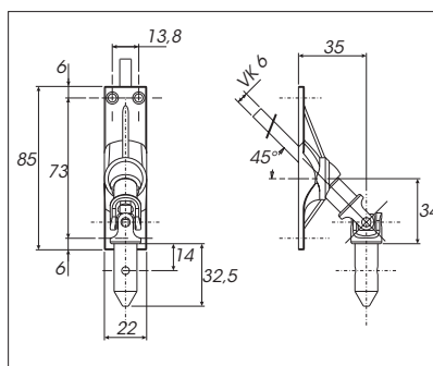
Fig. 10b : Doorvoer 45°
