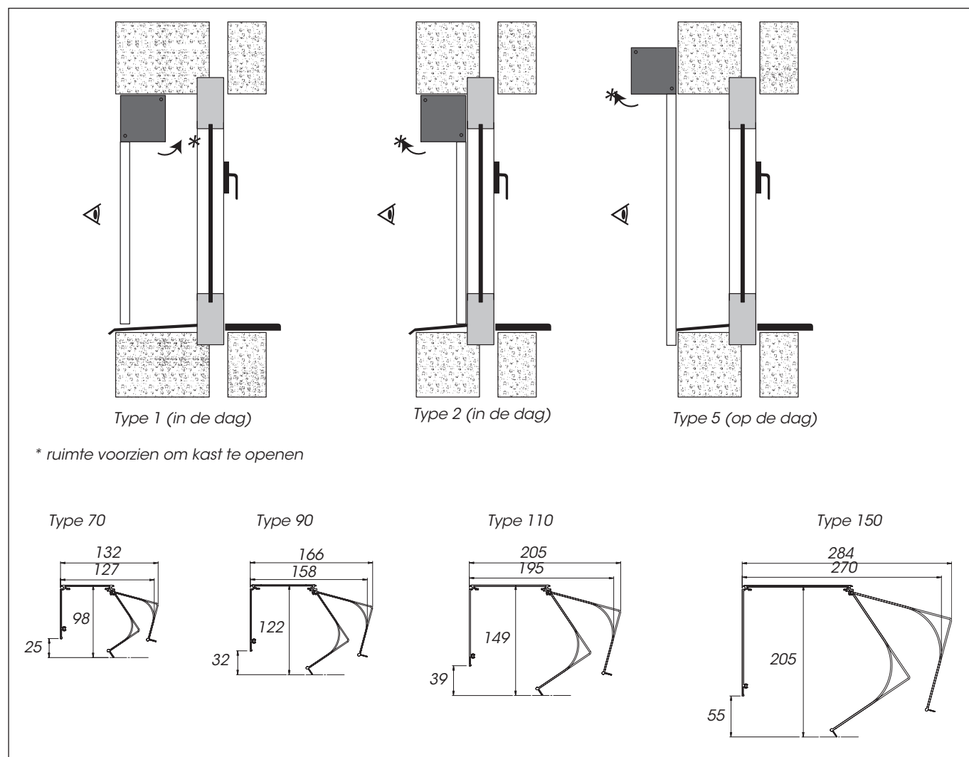
Fig. 9: Montagemogelijkheden
