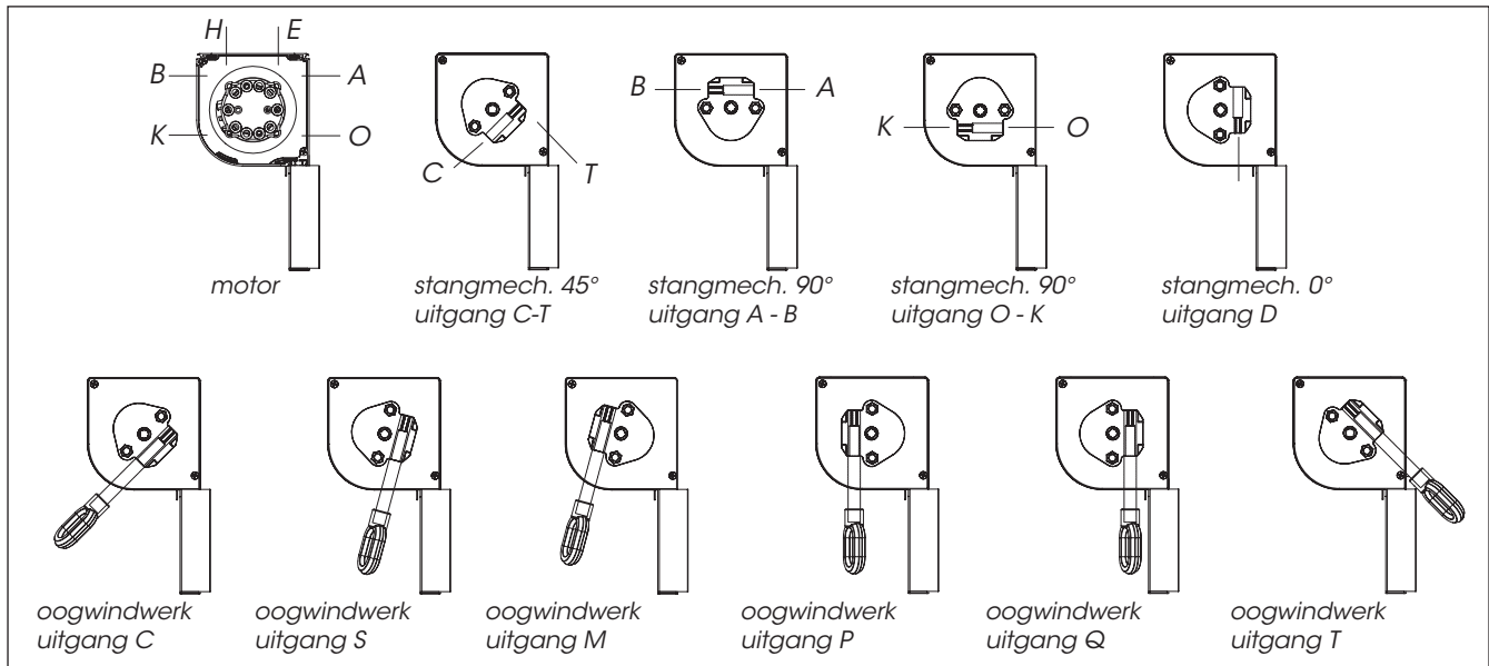
Fig. 11: Bedieningsuitgangen
