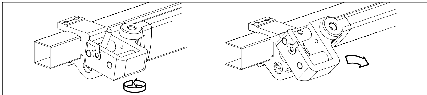
Fig. 6 : Angular displacement system
