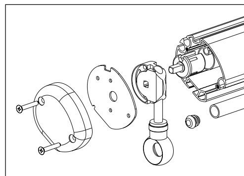
Fig. 19 : Variovalance
