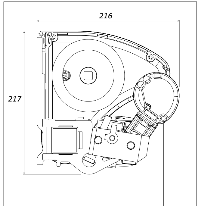
Fig. 3 : Section PR220
