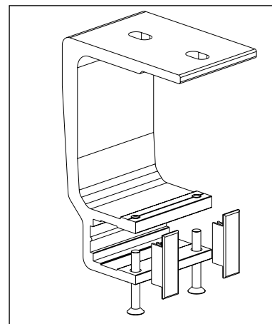
Fig. 10 : Ceiling bracket
