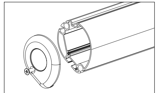
Fig. 4 : Round extension pole (standard)
