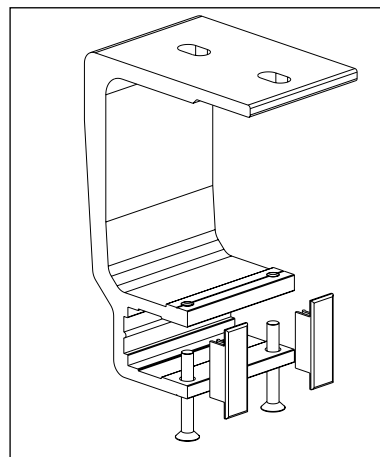
Fig. 10 : Plafondconsole
