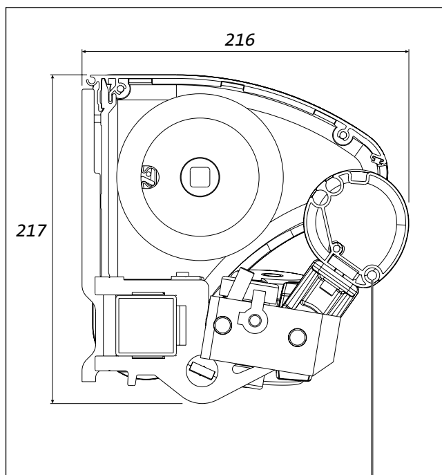
Fig. 3 : Doorsnede PR220
