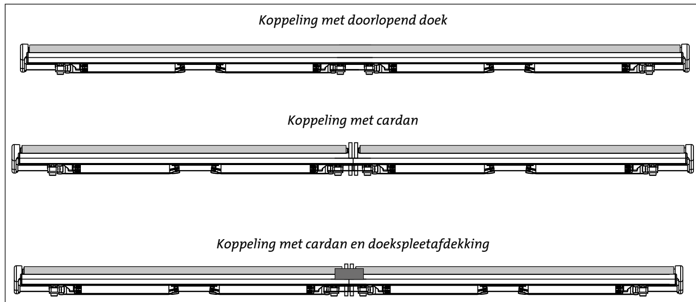
Fig. 14 : Koppelmogelijkheden
