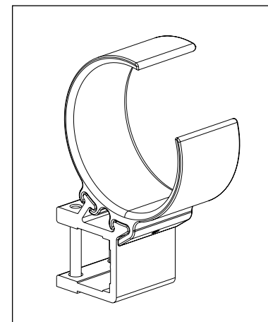
Fig. 12 : Doekrolondersteuning
