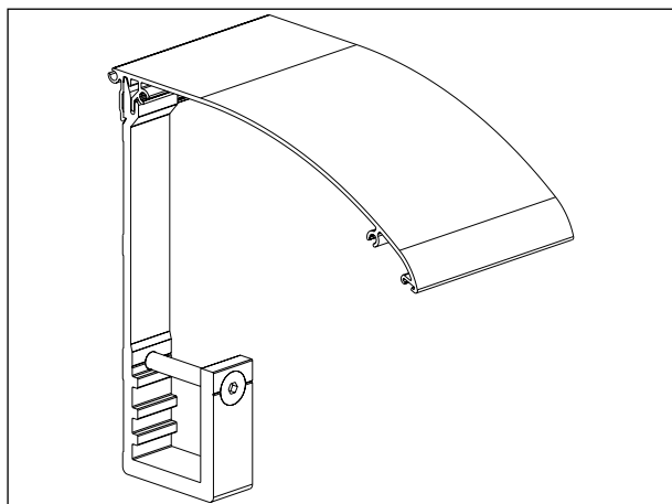
Fig. 8 : Kapondersteuning
