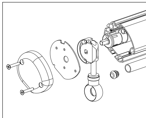
Fig. 19 : Variovolant
