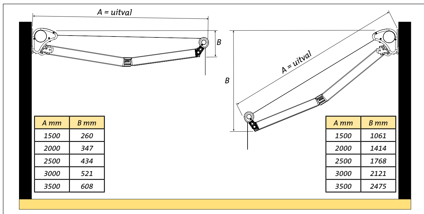
Fig. 17 : Minimale en maximale instellingen
