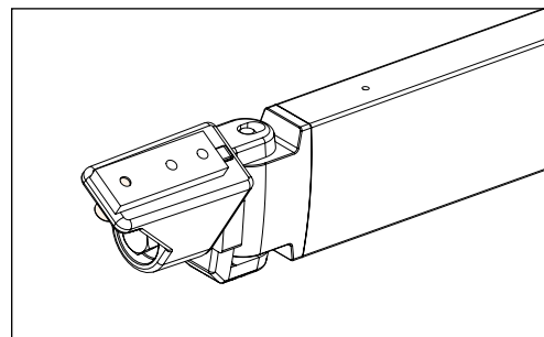
Fig. 7 : Voorlijstbevestiging
