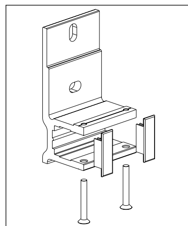
Fig. 9 : Muurconsole
