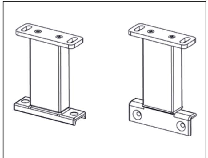
Fig. 9 : Supports prolongés
