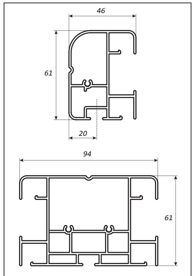
Fig. 1 : Coulisses
