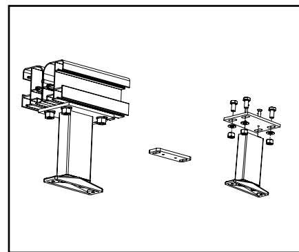
Fig. 15: placement soutien accru au milieu
