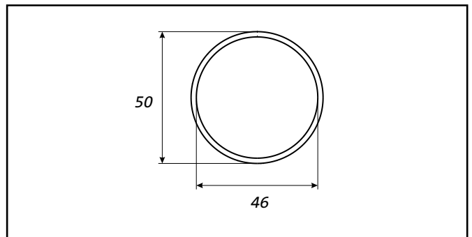
Fig. 5 : Le rouleau intermédiaire
