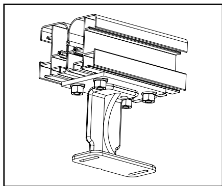
Fig. 13: support standard de placement VZ720 au milieu
