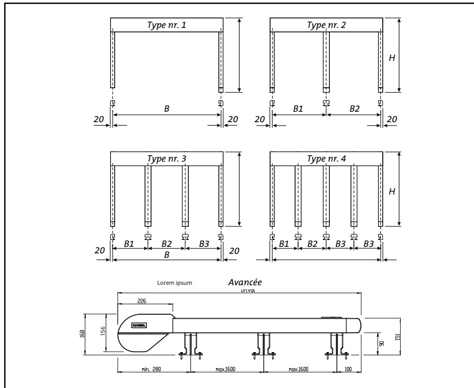
Fig. 16 : Mesurage et montage
