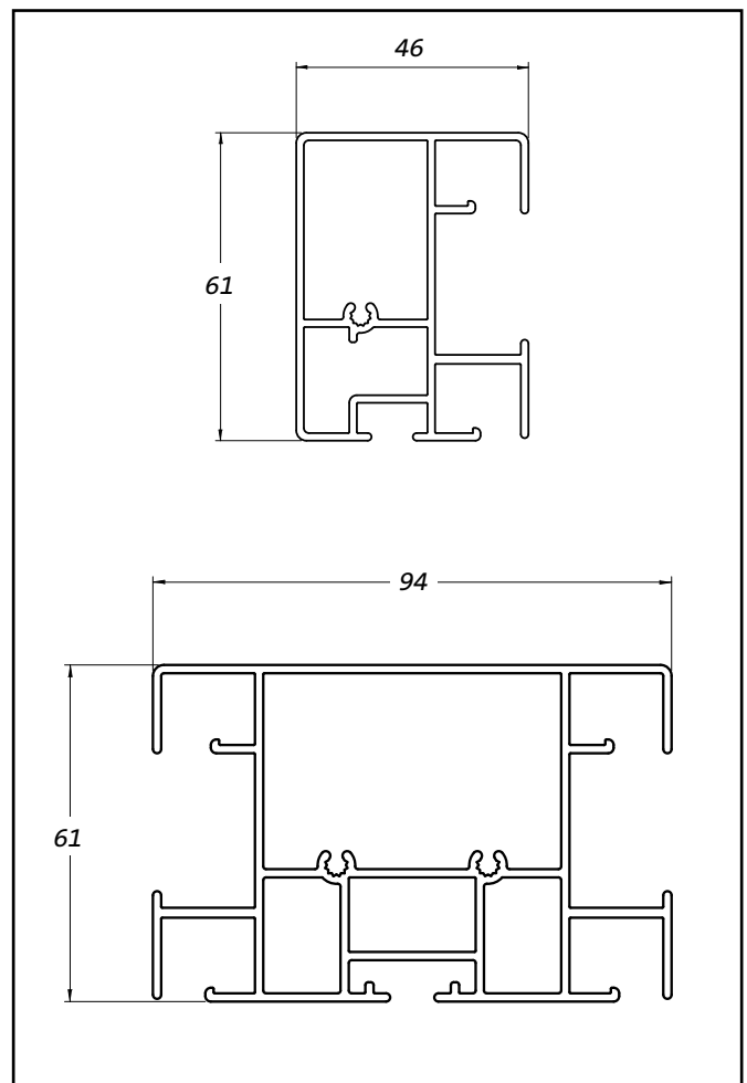
Fig. 1 : Les coulisses
