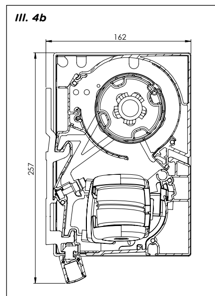
Figuur 4b : coupe du modèle BX270 + LED
