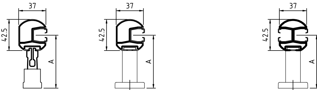
Enkelvoudige zijgeleiders (rond)
