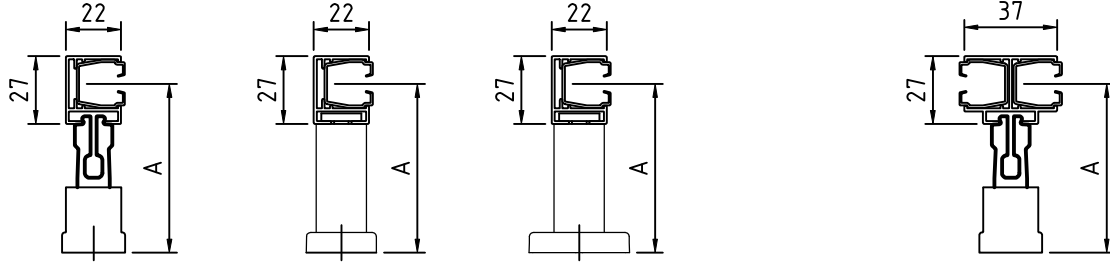
Enkelvoudige zijgeleiders 30x32 (voor zelfdragende systemen)
