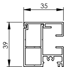
GUIDE
